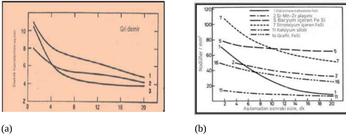
Şekil 2. a) Gri demirde ötektik hücre sayısında azalma b) küresel grafitli dökme demir malzemede küre sayısında azalma [5]
