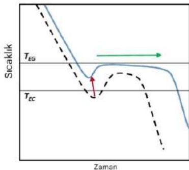
Şekil 1. Aşılamanın soğuma eğrisi üzerindeki etkisi [3]
