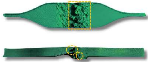
ABS Plus- ABS Plus, Deney 17 Çekme Dayanımı: 15.52 MPa
