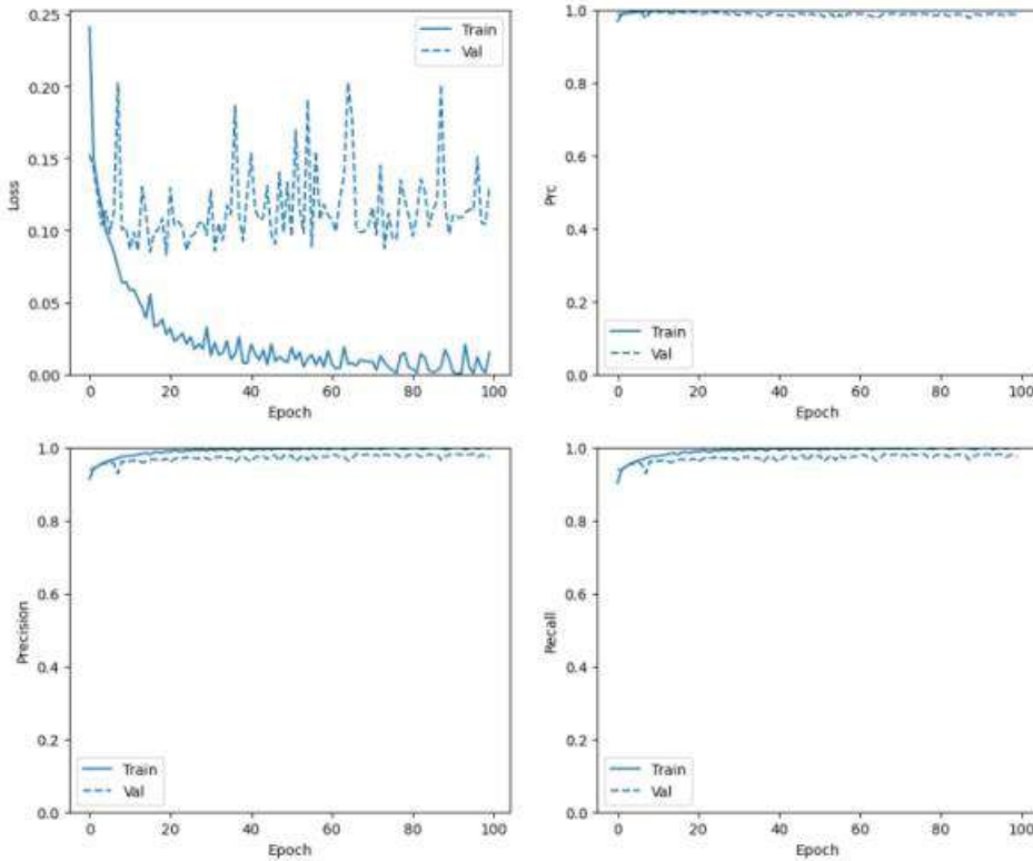
Şekil 6. MobileNet modelinin Loss, PRC, Precision, Recall eğrileri
