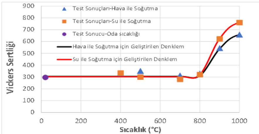
Şekil 9. AISI 440C çeliğinin farklı sıcaklıklarda ısıtıl işlem sonrası hava veya su ile soğutma durumlarına göre elde edilen sertlik değerleri ve geliştirilen pratik model
