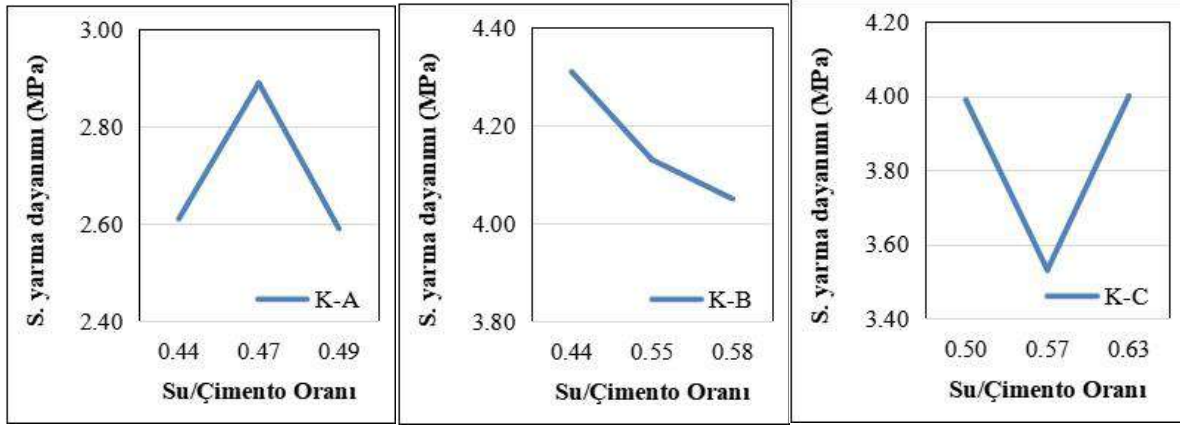
Şekil 6. Silindir yarma dayanımı değerlerinin su/çimento oranlarına göre değişimleri
