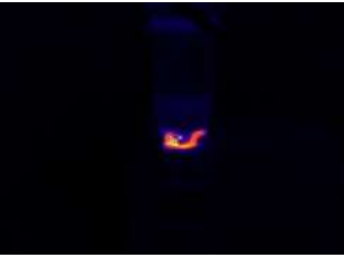
PA6 GF30 - PA6 GF30: Üçgen uç 40 mm/dak, 2250 dev/dak, 189.20°C
