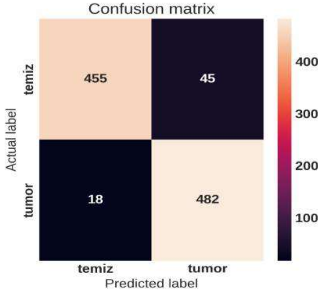
Şekil 3. EfficientV2B0 modeline ait karmaşıklık matrisi.
