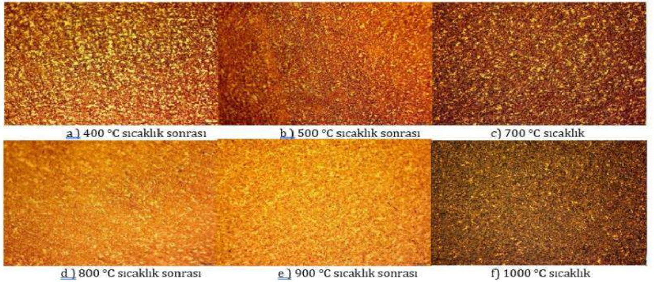
Şekil 8. Farklı sıcaklıklarda ısıtıl işlem görüp, su ile soğutulan test numunelerinin dağlama sonrası görüntüleri
