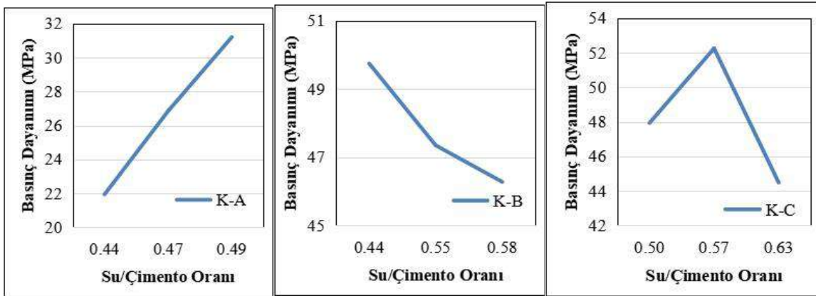
Şekil 4. Küp numune basınç dayanımlarının su/çimento oranlarına göre değişimleri
