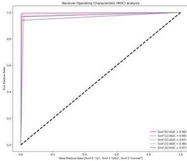
Şekil 7. MobileNet modelinin ROC eğrisi değerleri
