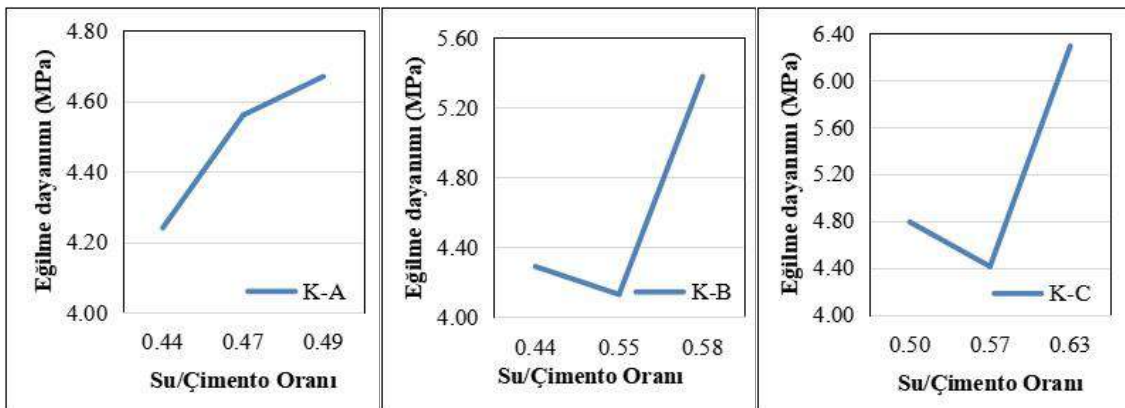
Şekil 5. Eğilme dayanımı değerlerinin su/çimento oranlarına göre değişimleri
