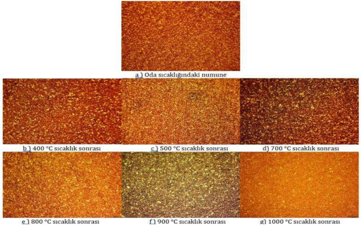
Şekil 7. Farklı sıcaklıklarda ısıtım işlemi görüp, hava ile soğutulan test numunelerinin dağlama sonrası görüntüleri
