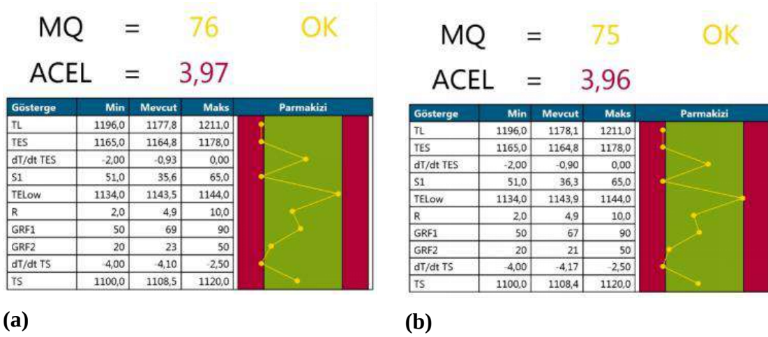
Şekil 7. Termal analiz verileri ve optimum aralık değeri. a) Boş (Aşırsız) numune b) %0,4 Yeşil SiC içeren numune
