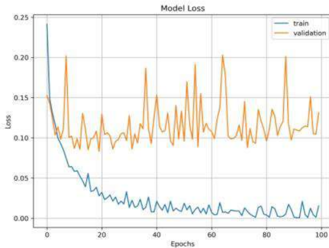
Şekil 4. MobileNet modelinin kayıp değeri grafiği
