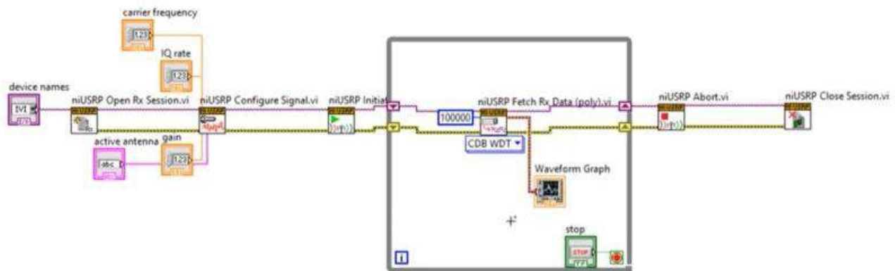
Рисунок 3. Блок-схема приемного тракта
