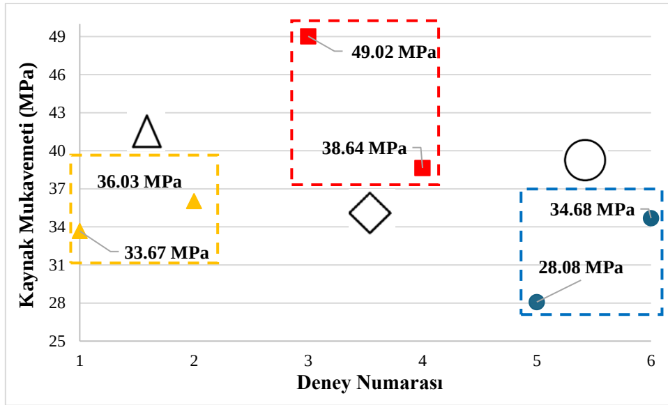
Şekil 12. PA6 GF30-PA6 GF30 plakalarda kaynak mukavemetleri.
