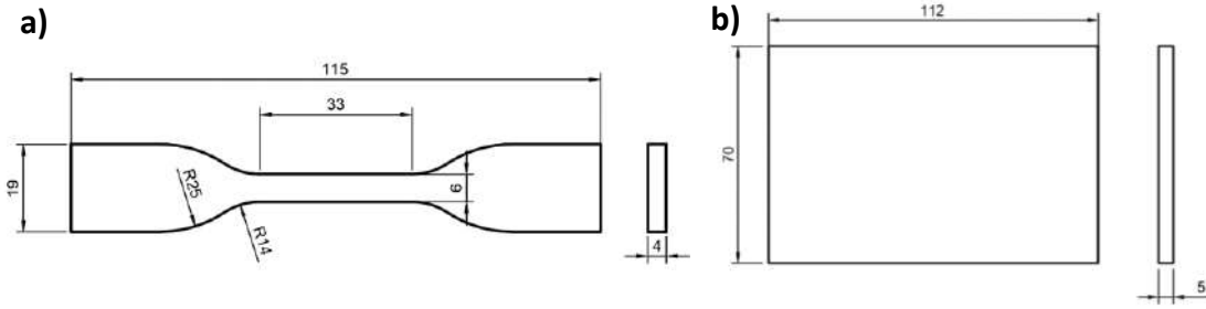
Şekil 2. Üretilen numunelerin teknik çizimleri (tüm boyutlar mm cinsindendir).
