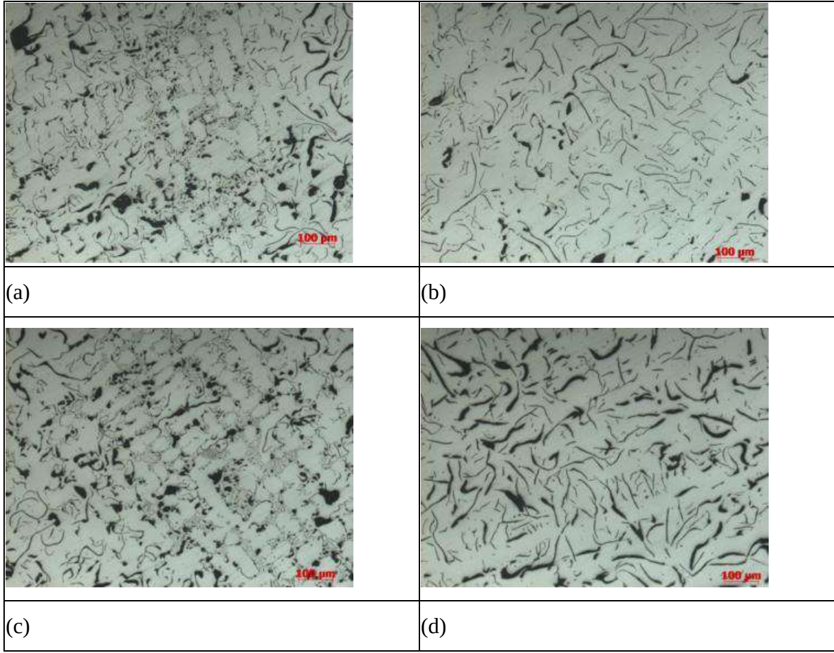
Şekil 8. Test edilen numunelerinin mikroyapısı a) Aşısız (kenar kısım) b) Aşısız (orta kısım) c) Aşılı (kenar kısım) d) Aşılı (orta kısım)
