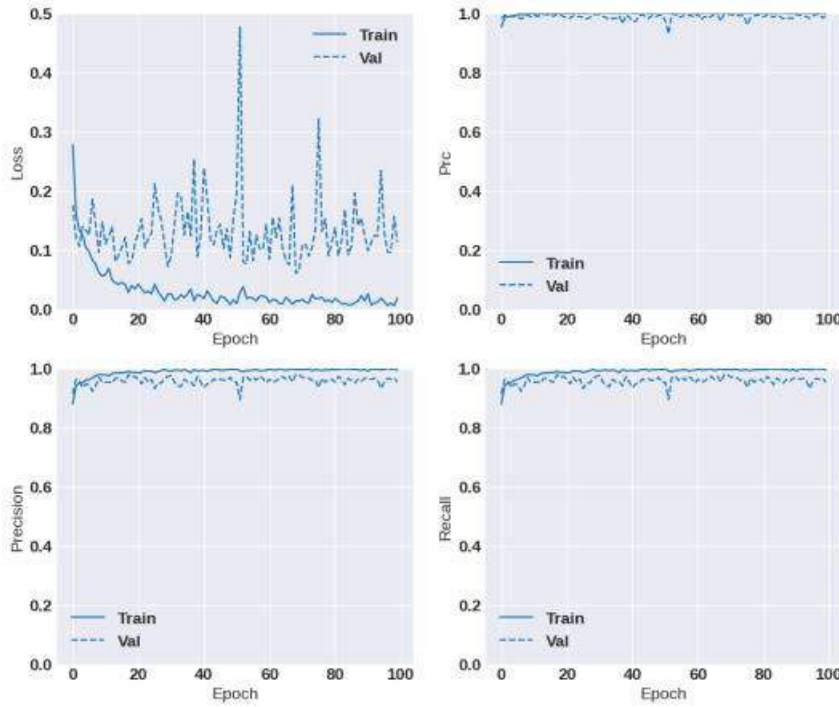
Şekil 5. EfficientV2B0 precision, recall, PRC ve loss eğrileri.
