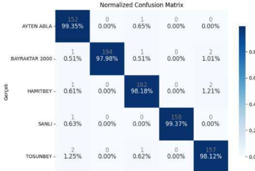
Şekil 4. ResNet101 modelinin karmaşıklık matrisi.
