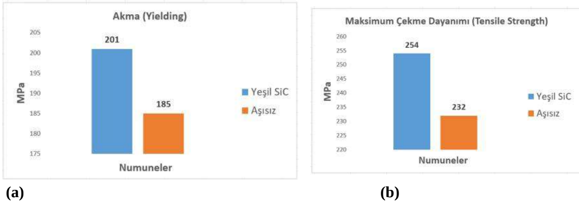
Şekil 10. Numunelerin maksimum çekme ve akma dayanımı değerleri
