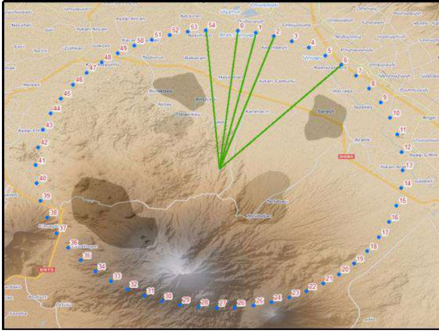
Şekil 19. HDF_AĞRI hedefinin İHA ile kesintisiz görülebildiği hatlar (Senaryo 10)
