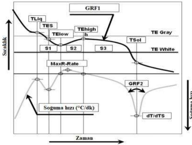
Şekil 5. Termal analiz sonucu çizilen soğuma eğrisi ve bazı değerlerin eğri üzerinde gösterimi
