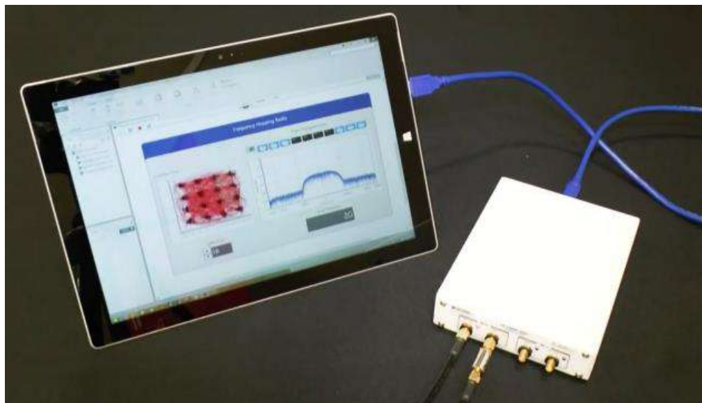
Рисунок 5. Подключение NI USRP к планшету (к хосту)
