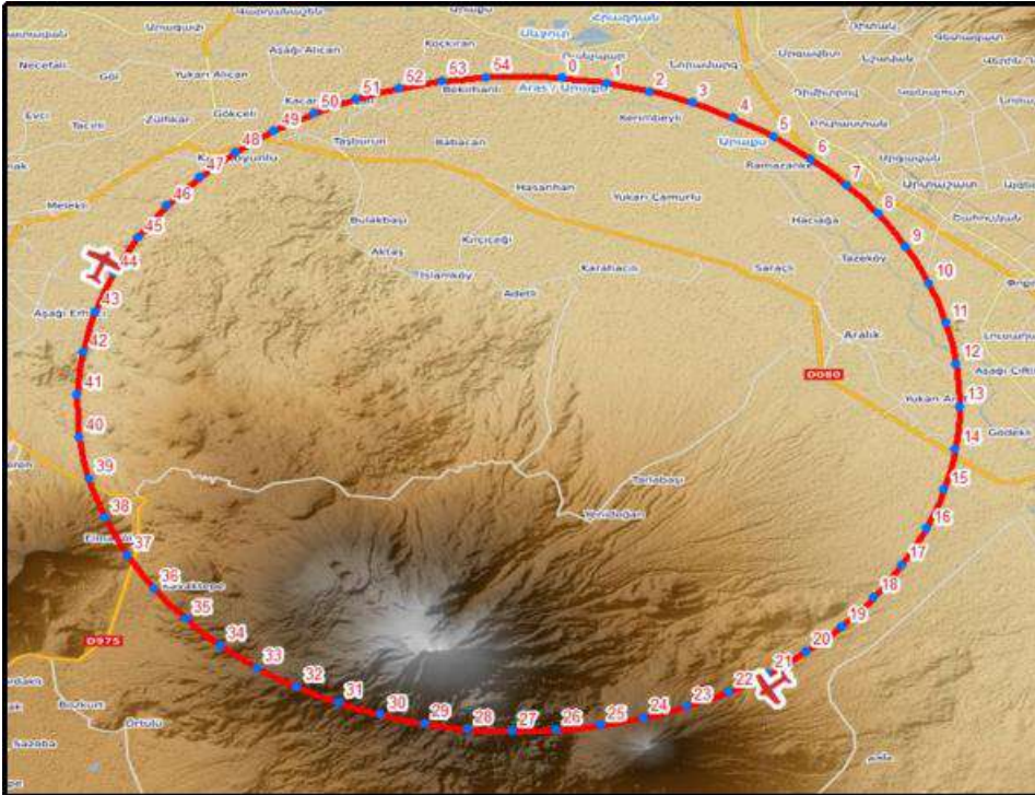
Şekil 8. HDF_AĞRI İHA rotası üzerinde oluşturulan noktalar ve İHA konumu
