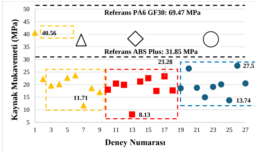
Şekil 11. ABS Plus- PA6 GF30 plakalarda kaynak mukavemetleri.
