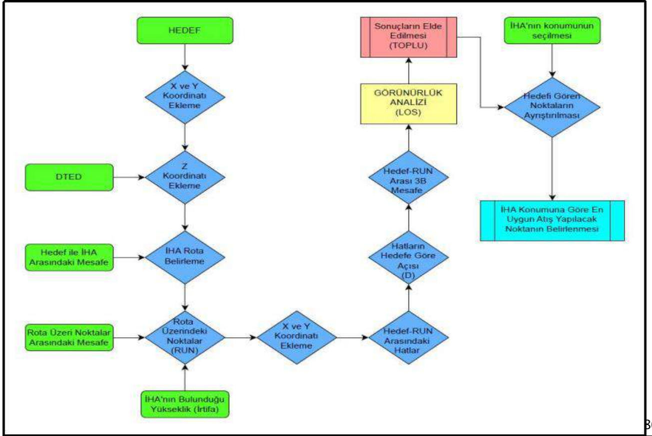
Şekil 6. Görünürlük analizi akış diyagramı
