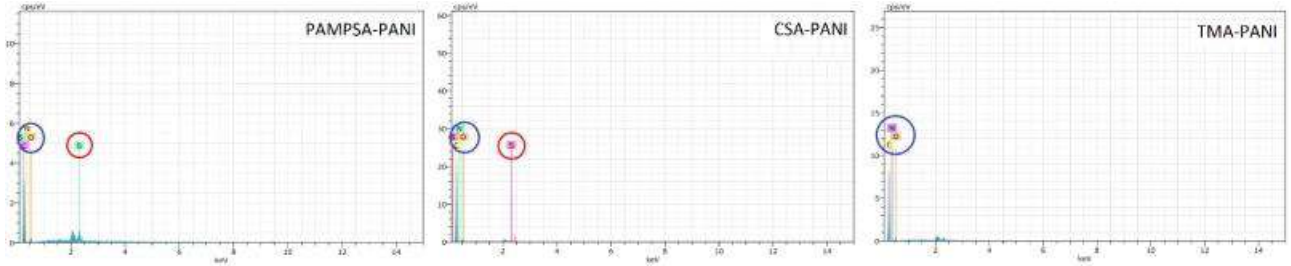
Şekil 6. Hazırlanan polimerlere ait EDX sonuçları
