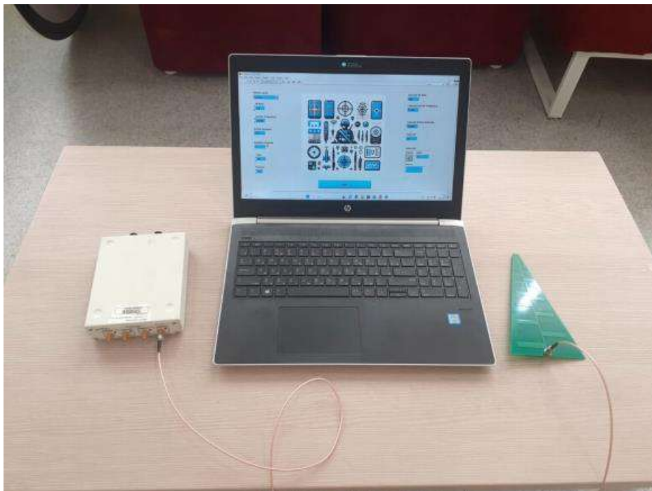
Рисунок 2. Макет устройства радиоэлектронного подавления (подключена логопериодическая патч-антенна)
