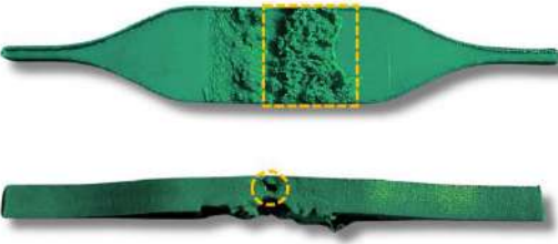
ABS Plus- ABS Plus, Deney 25 Çekme Dayanımı: 15.08 MPa
