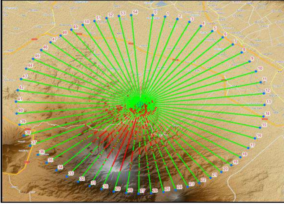
Şekil 10. HDF_AĞRI isimli hedefe göre görünürlük analizi sonucu (Senaryo 1)
