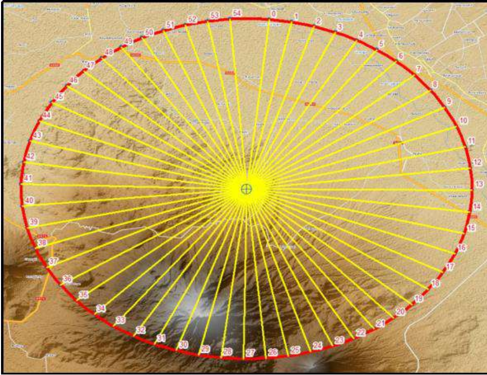
Şekil 9. HDF_AĞRI ile İHA rotası üzerindeki noktalar arası hatlar
