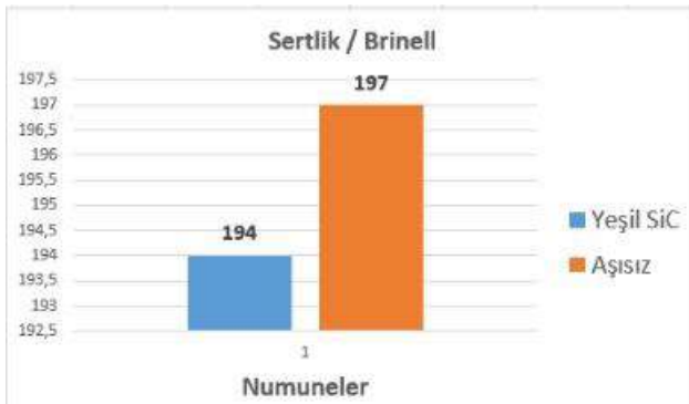
Şekil 9. Numunelerin ortalama sertlik değerleri
