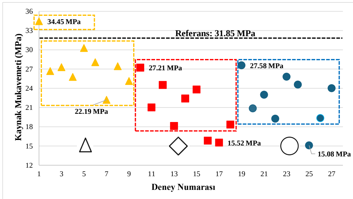
Şekil 10. ABS Plus-ABS Plus plakalarda kaynak mukavemetleri.
