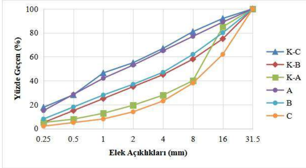
Şekil 1. Kırmataş agregalara ait elek analizi deney sonuçları
