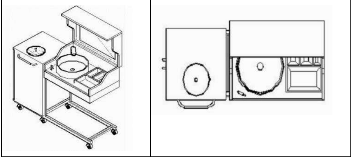
Şekil 2. Mobil kişisel bakım ünitesinin izometrik görünümü
