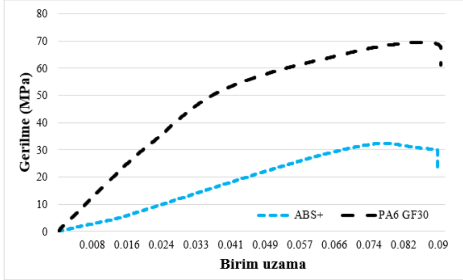
Şekil 5. ABS Plus ve PA6 GF30 gerilme-birim uzama grafiği
