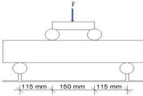
Şekil 2. Eğilme dayanımı deneyi şematik görseli
