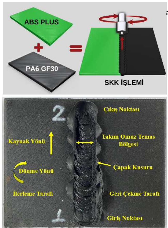
Şekil 4. SKK işleminin şematik gösterimi (a) ve temel kavramlar (b).
